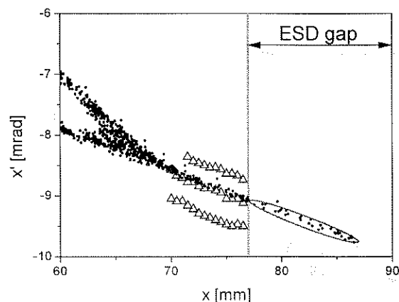
図5：静電デフレクター入口での位相空間の様子。測定結果（三角）とシミュレーション（黒点）。
