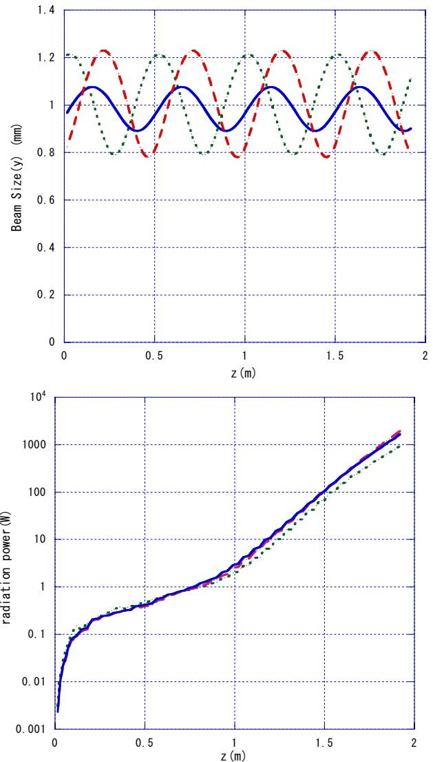
図2：鉛直方向のビームサイズ(上)と光のパワー(下)
