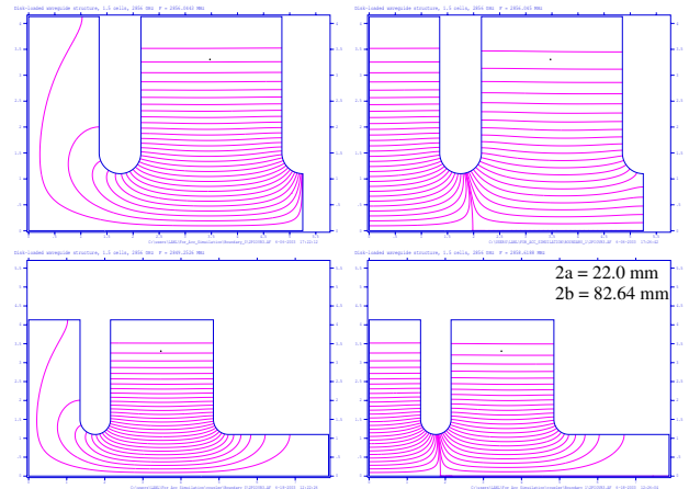
図 1: POISSON SUPERFISH で計算した加速管内電場。左上：ノーマルセクション Neumann Boundary、右上：ノーマルセクション Dirichlet Boundary、左下：入出力カップラ Neumann Boundary、右下：入出力カップラ Dirichlet Boundary。
