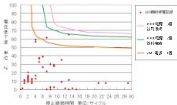
図4：VME直流電源耐力テスト結果
