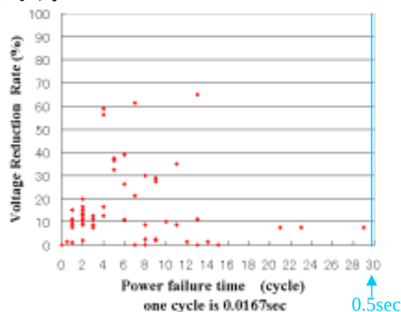
図.1 過去5年間にSPring-8で発生した電力トラブル。縦軸は、電圧低下度。横軸は、電力トラブル継続時間である。時間は1/60秒 = 1 cycleである。
