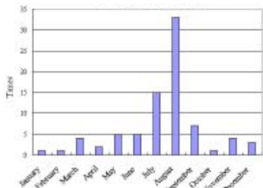
図2：月別の瞬時電圧低下の統計
