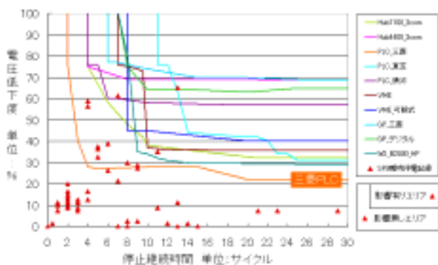
図3：機器の瞬時電圧低下耐性テスト結果
