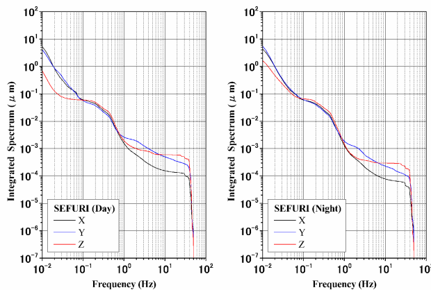
図-5 脊振地点：昼夜別積分パワースペクトル
