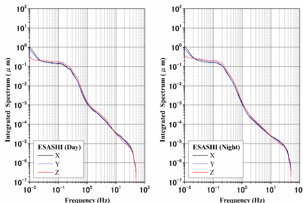
図-7 江刺地点：昼夜別積分パワースペクトル
