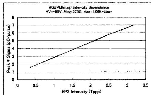
図5 ビーム強度を変化させたときの信号強度の変化。横軸は取り出しビームの強度 ( 10^{12} proton / spill)
