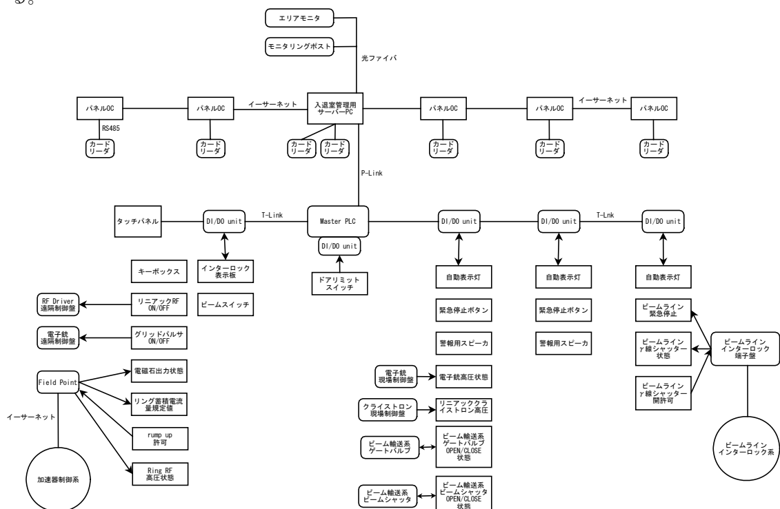
図3：放射線インターロック系機器構成概念図
