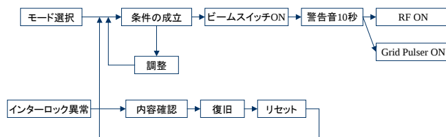
図2：ビーム出射の動作フロー
