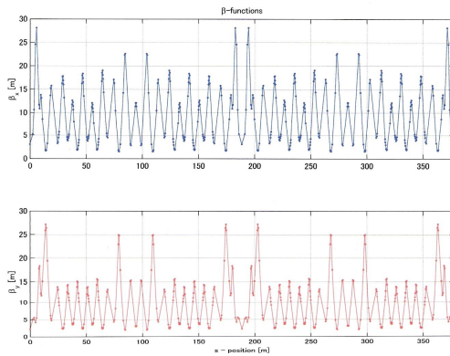
図3 AR 2回対称オブティクス
