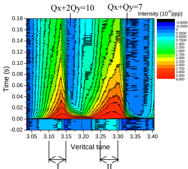
図4 バンチビームのときのチューンサーベイによる強度の時間経過および垂直方向動作点依存性
