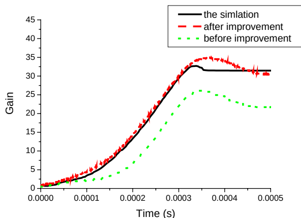
図2 最適化前後とシミュレーションによる入射ゲインの比較（実線：シミュレーションによる入射ゲイン、破線：最適化後の入射ゲイン、点線：最適化前の入射ゲイン）
