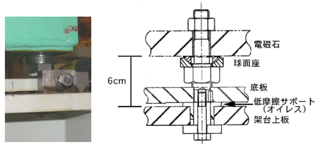
図2. 電磁石の架台への固定部
