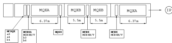
図1 LHC衝突点でのビーム収束系
