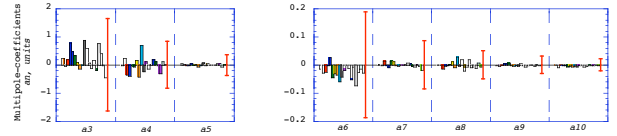
図 5 MQXA19 台の a_n 成分と許容値
