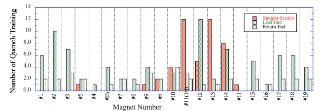
図4 MQXAのクエンチ発生場所
