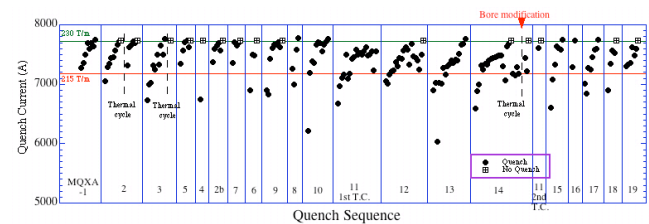
図3 MQXAのクエンチ特性
