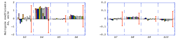
図 6 MQXA19 台の b_n 成分と許容値
