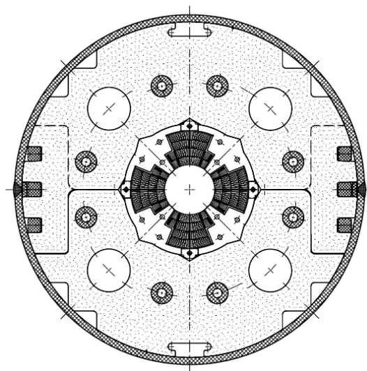
図2 MQXA断面形状
