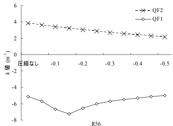
図4：図2中のQF1とQF2のk値の変化
