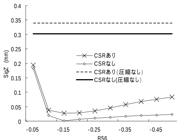
図5： R_{56} と13m直線部の \sigma_z の関係
