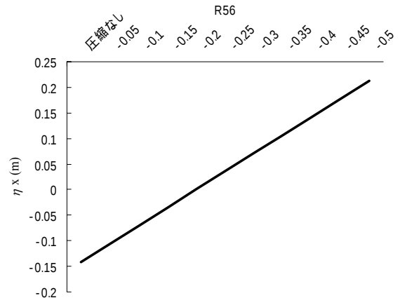
図3：周回部中央の分散関数 \eta_x と R_{56} との関係
