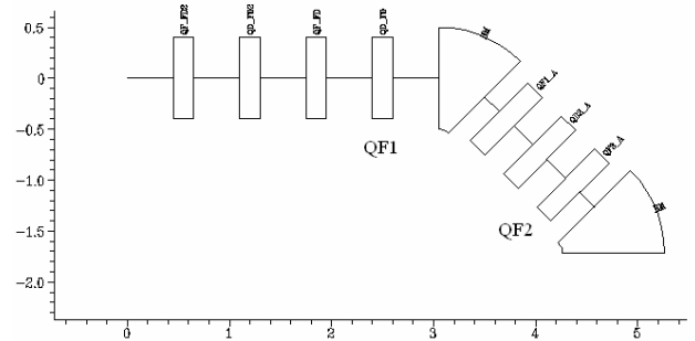
図2：周回部のデザイン
