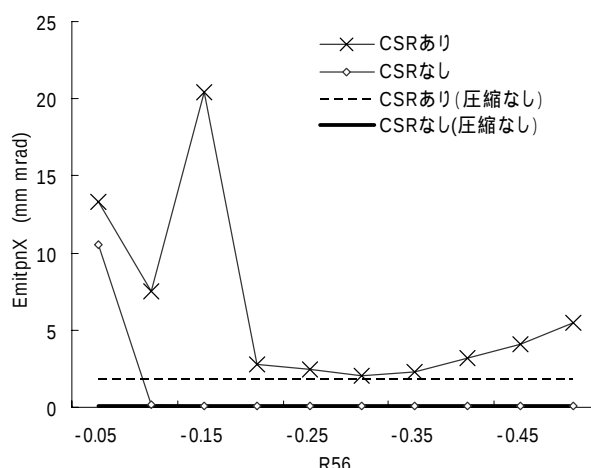
図6： R_{56} と13m直線部の \varepsilon_{nx} の関係
