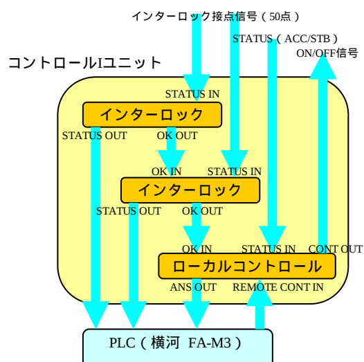
図1：コントロールユニットの入出力信号
