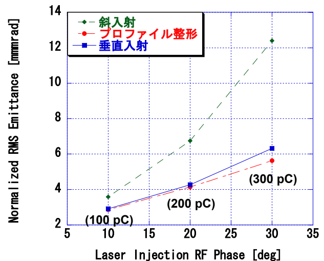
図6：エミッタンス測定結果
