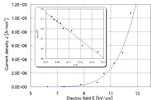
図 2. CNT電界放出特性試験結果。図中にはFowler-Nordheimプロットを挿入した。曲線はフィッティングの結果を示す。陰極-陽極間距離4mm。実験時の真空度10 -6 ~10 -7 Torrであった。
