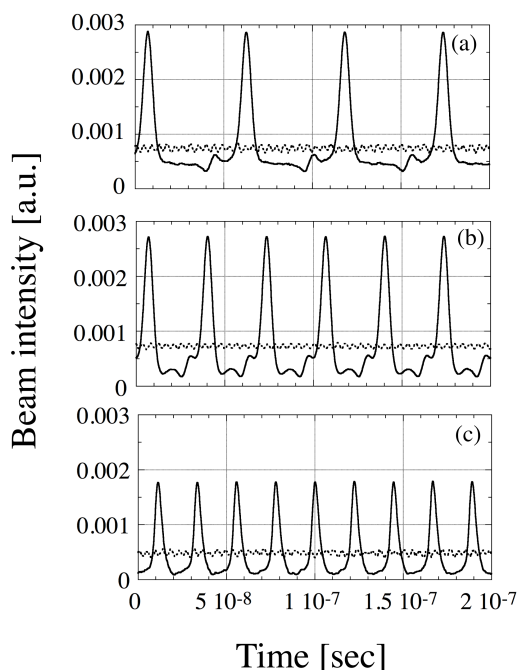
図7：FC2で測定されたパンチ波形の例。ビームの種類と rf 周波数は、(a) \text{Ar}^{8+} ビーム/ 18\text{MHz} 、(b) \text{O}^{5+} ビーム/ 30\text{MHz} 、(c) \text{H}^{+} ビーム/ 45\text{MHz} である。実線と点線は高周波電力のON( 0.1\text{kV} )とOFFに対応している。
