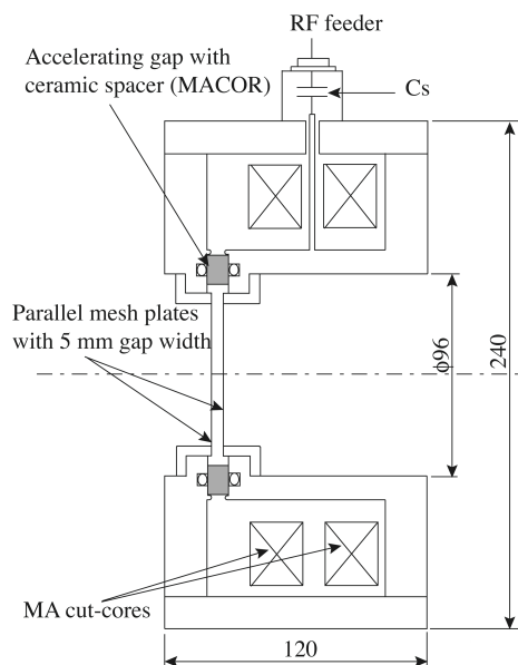
図1：空洞断面図
