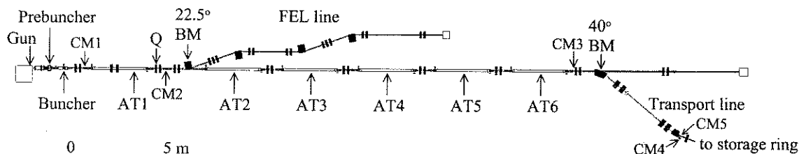
図 1: リニアックの全体図. AT は加速管を示す.
