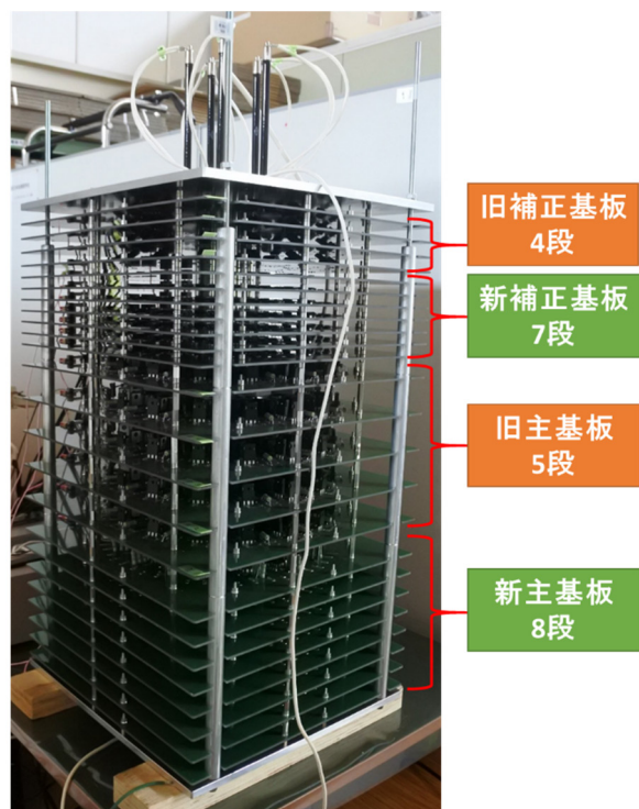
基板積み上げ外観 (主基板13枚、補正基板11枚)
