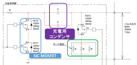
新主基板ブロック図 (主回路部)
