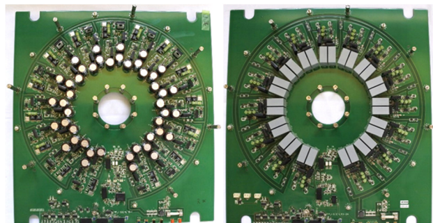
旧主基板
