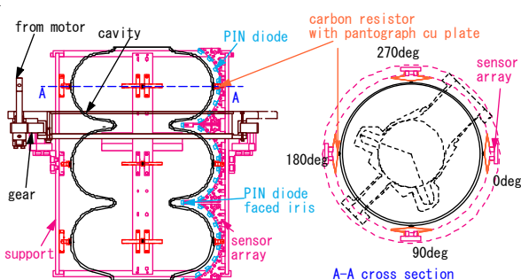
図4：回転マッピング装置の詳細図。水色がPIN diodeの配列。橙色がバネ付きの炭素温度計。
