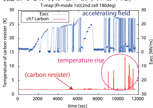
図7：7回目の2セル 180-240^\circ での温度上昇。
