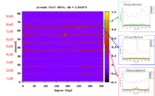
図8：7回目加速モードのX線マッピング測定結果。右図は各セルでの1次元トレース。
