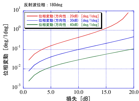
図8. 損失の変化による位相補償の変動
