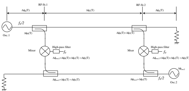
図2. 実際の回路構成、Case-1
