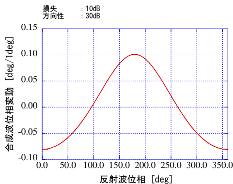
図7. 反射波の位相に対する補償回路の位相変動 (Case-3について)
