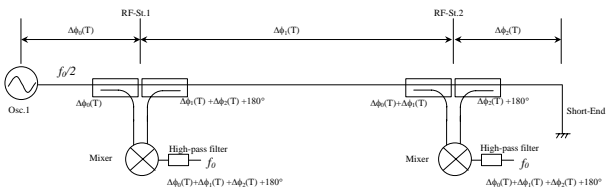
図4. 実際の回路構成、Case-3
