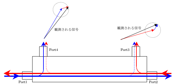
図5. 方向性結合器の方向性
