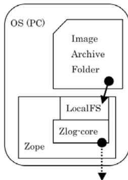
図2: 真空機器管理用Zlogの画像表示の仕組み (LocalFSを使用し、OS上のファイルをZopeのオブジェクトとして公開している)
