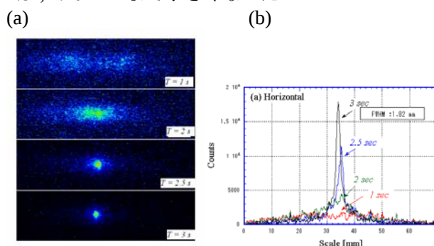
図8. 6 MeV/u の \text{Ar}^{18+} (粒子数 1 \times 10^6 )の電子冷却
