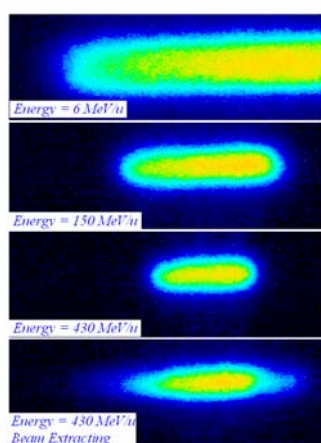
図7. 入射から取り出しまでの ^{12}\text{C}^{6+} の加速ビーム
