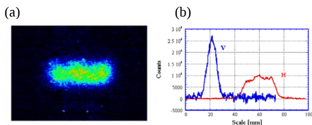
図6. ^{12}\text{C}^{6+} の単バンチのビームプロファイル
