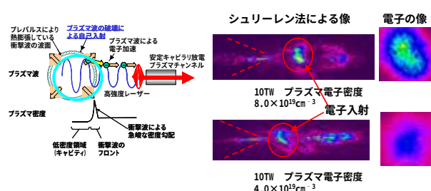
図7. 動的制御によるエネルギー単色化
