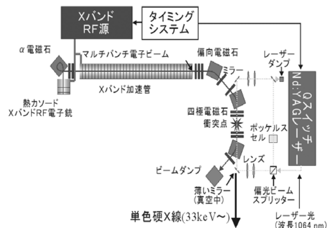
図4. 単色X線生成実証用Xバンドビームライン
