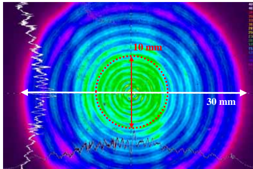
図 6 : レーザー光プロフィール
