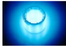
ガンマ線源からのチェレンコフ光
